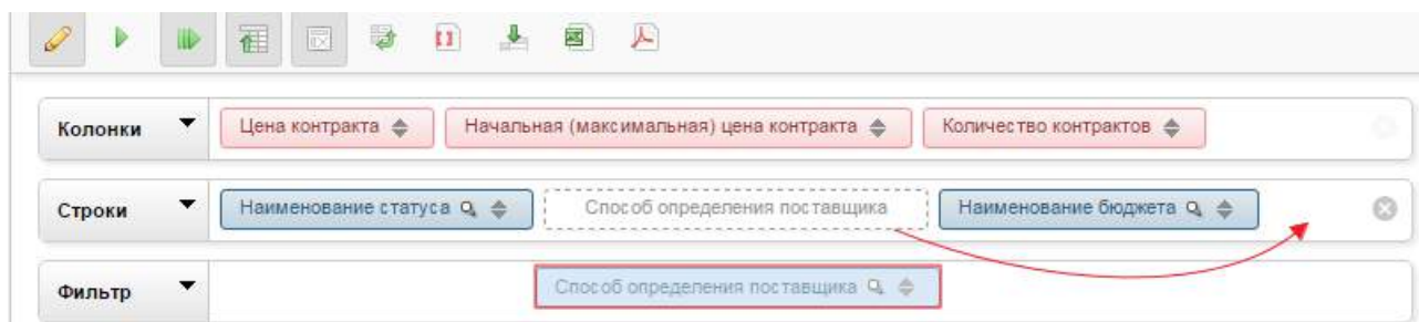
Рис. 7. Изменение расположения колонки/строки
