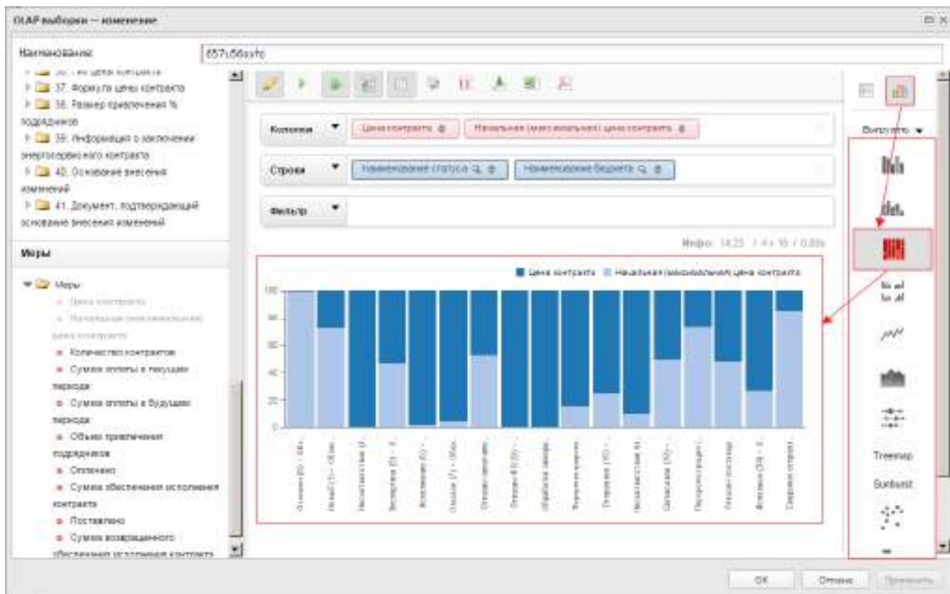
Рис. 12. Отображение данных в режиме диаграммы «Гистограмма 100%»
